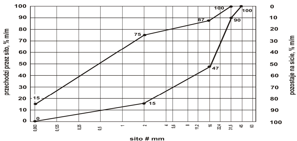
Rys. 4. Uziarnienie mieszanki niezwiązanej 0/31,5 dla nawierzchni
